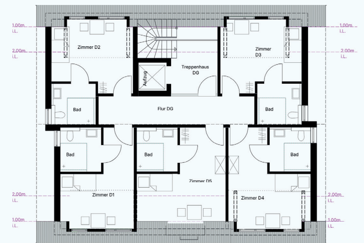
Dachgeschoss
