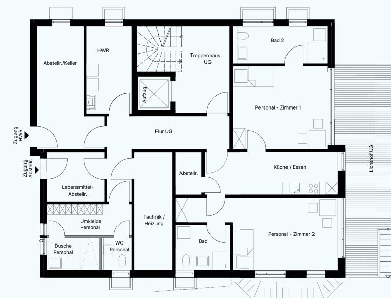
Untergeschoss
