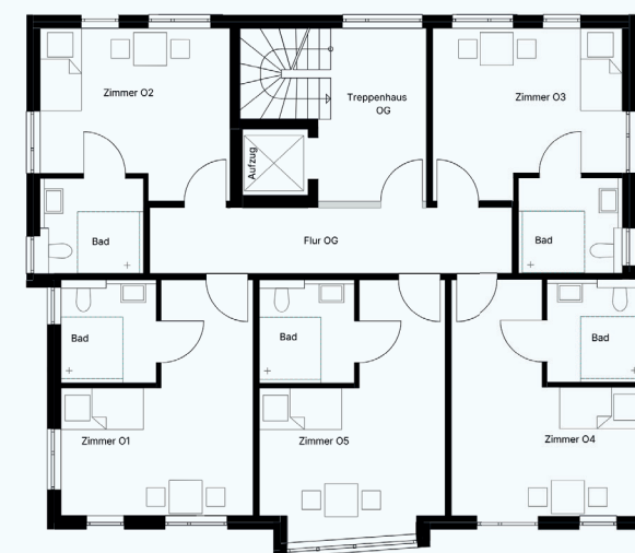
Obergeschoss
